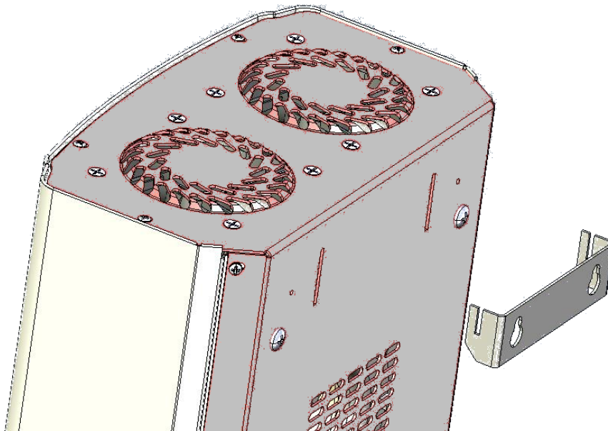
Рисунок 4. Кріплення стабілізатора на установчу планку
