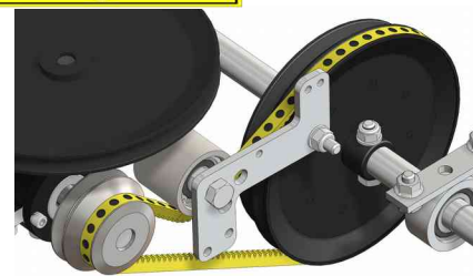
Obr. 24: Rychlost nižší
