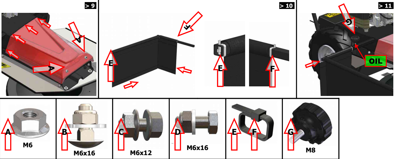
Obr. 3: Sestavení stroje
