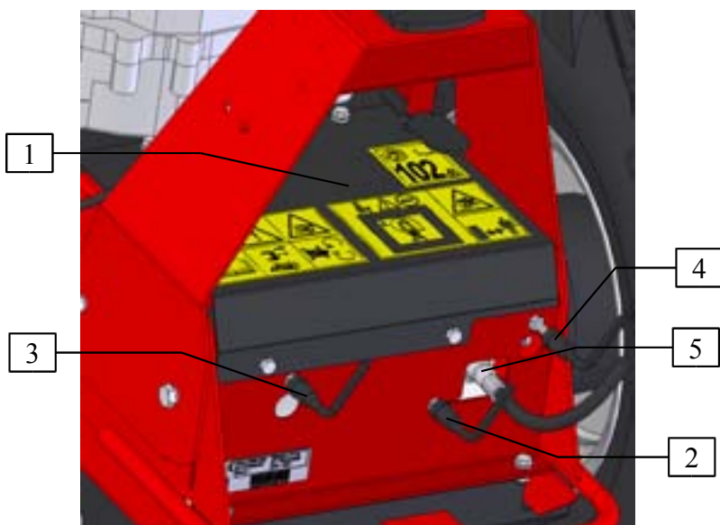
Obr. 12: Seřizovací šrouby napinacích kladek
