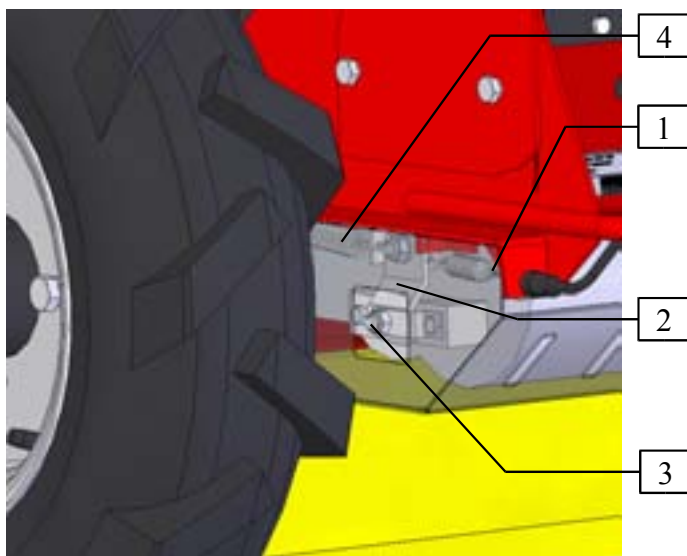
Obr. 14: Seřízení automatické brzdy pojezdu
