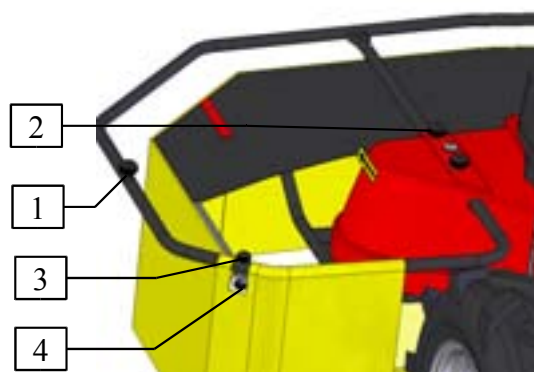
Obr. 5: Uchytení ochranné plechy zezadu
