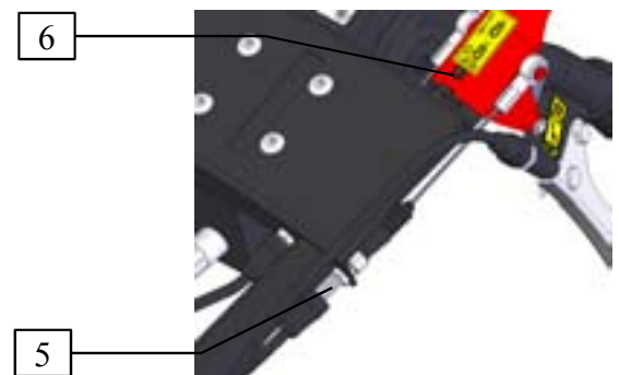
Obr. 15: Seřizovací šroub automatické brzdy pojezdu
