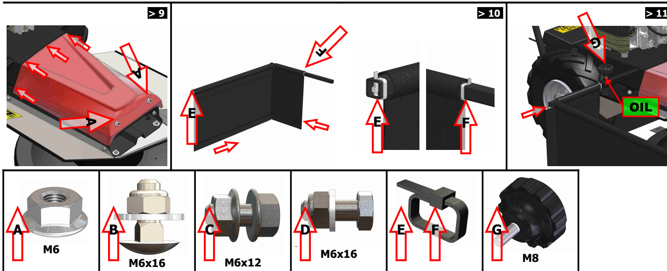
Obr. 3: Sestavení stroje
