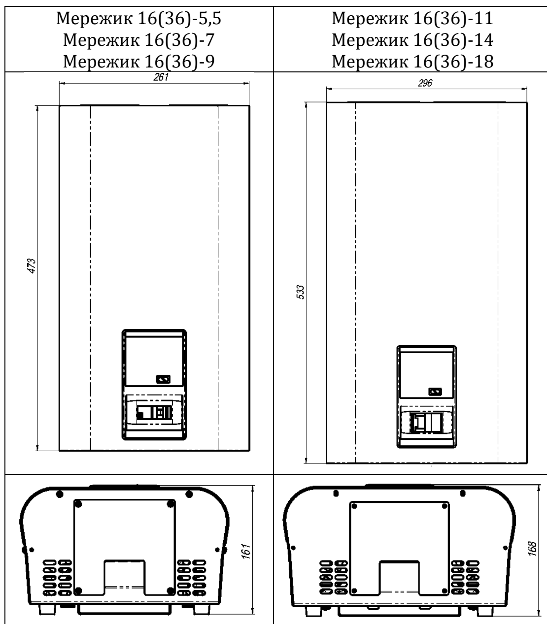
Рисунок 6. Габаритні розміри стабілізаторів
