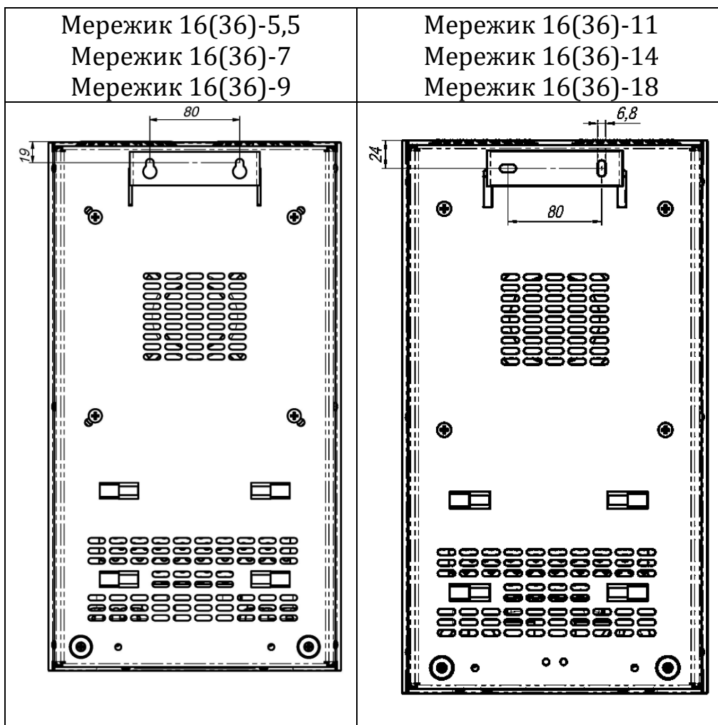
Рисунок 5. Установчі розміри стабілізаторів
