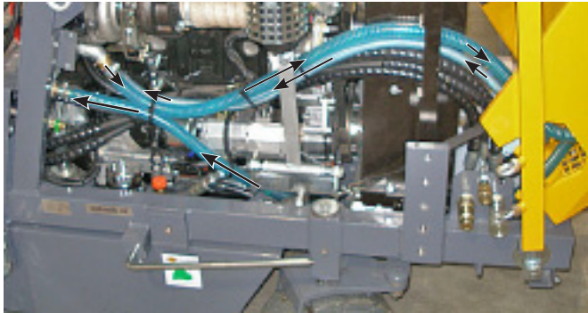
CF-6020 справа, подача воды к запорному крану (капот двигателя открыт) Рис. 5.15
