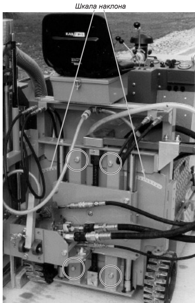
Шестигранные винты на режущей консоли
