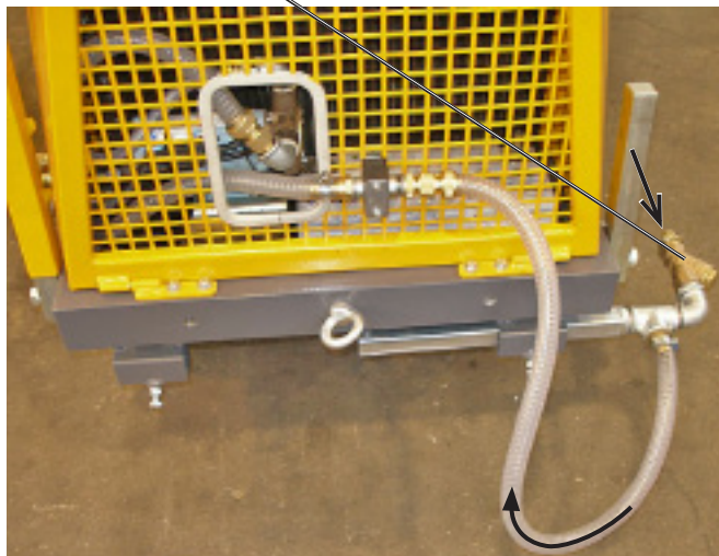
CF-6020 спереди, консоль смонтирована слева
