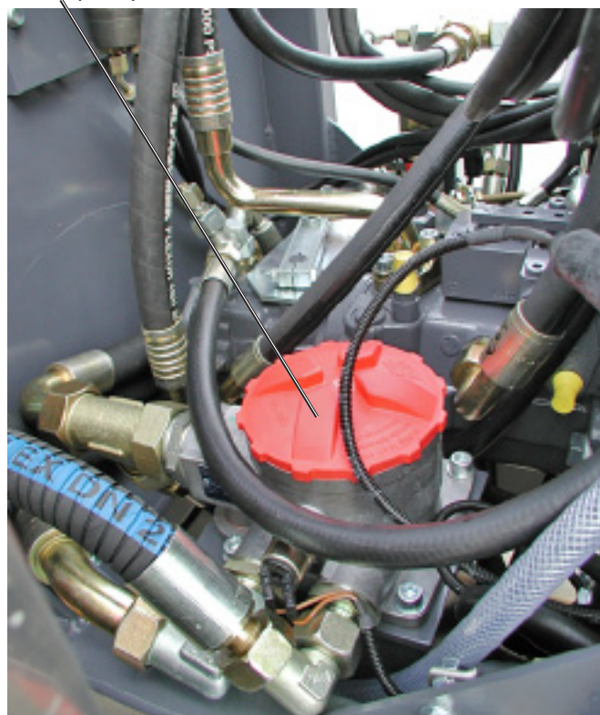
CF-6020 место оператора (справа), защитная крышка подножки снята
