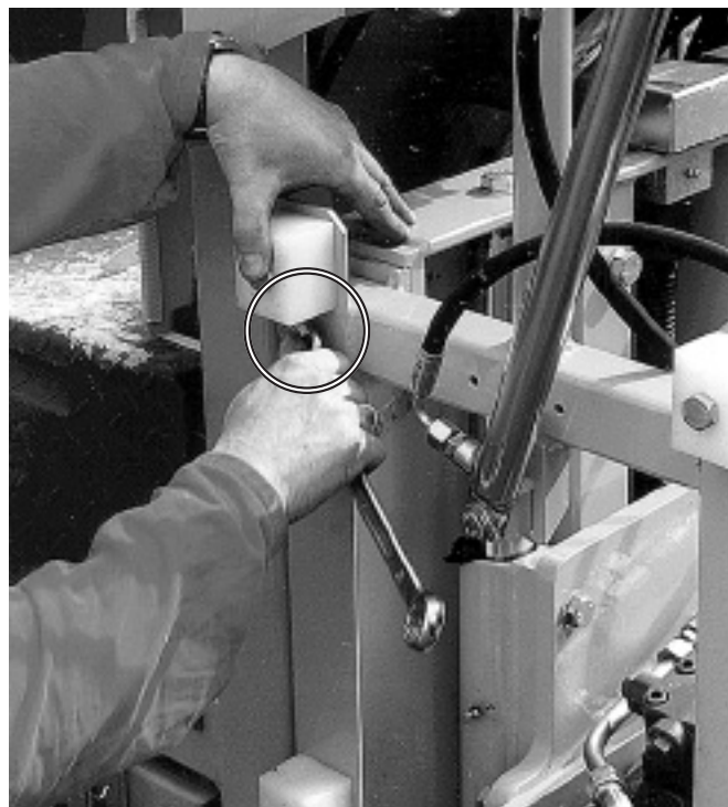
Снятие держателя защитного кожуха Рис. 7.3
