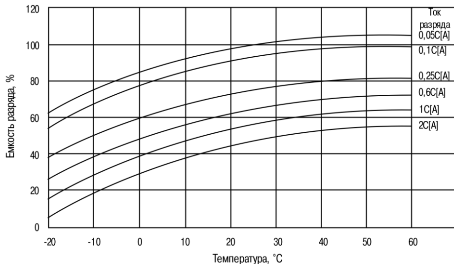
Рис. 6. Влияние температуры на емкость аккумулятора
