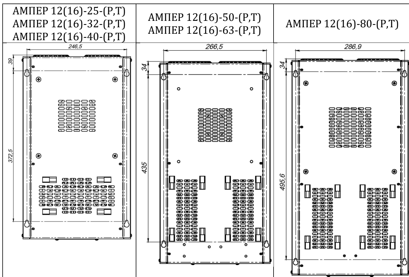
Рисунок 4. Установочные размеры стабилизаторов
