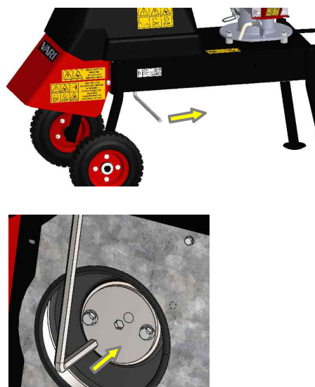
Obr. 7: Uvolňovací páka
