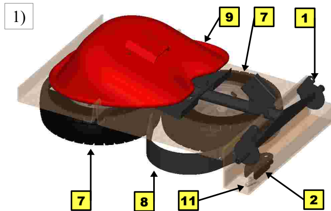
Obr. 2: Sestavení sulky
