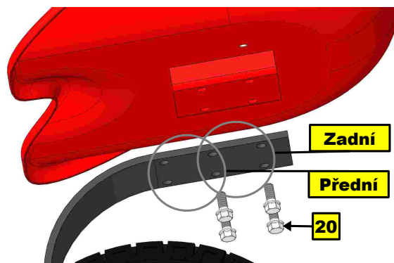
Obr. 5: Polohy sedačky
