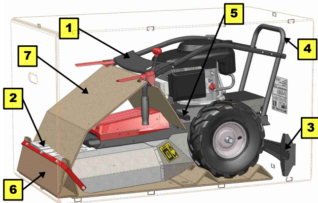
Obr. 1: Vybalení stroje
