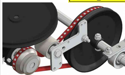
Obr. 23: Rychlost vyšší
