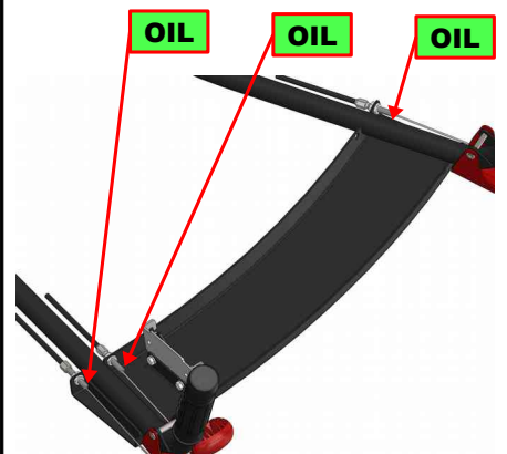
Obr. 7: Mazací místo
