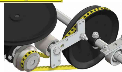
Obr. 24: Rychlost nižší
