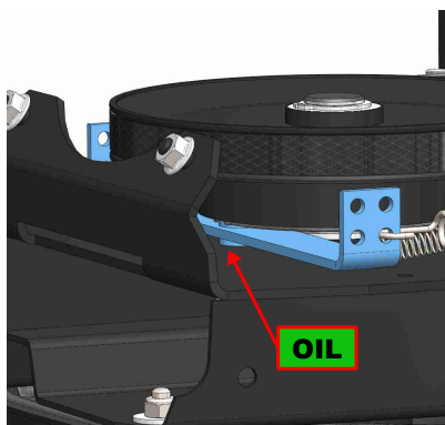
Obr. 9: Mazací místo
