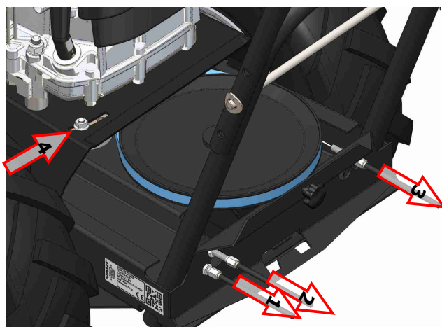
Obr. 10: Seřízení napínacích kladek pojezdu
