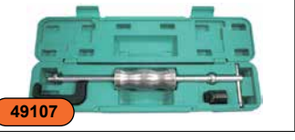
Съемник форсунок дизельных двигателей MB CDI AI020125
