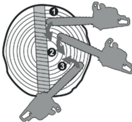
Рисунок 14. Схема розпилування колоди із використанням зубчастого упору бензопили.
