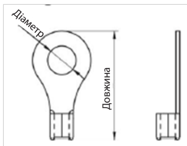
Кільцева клема:
