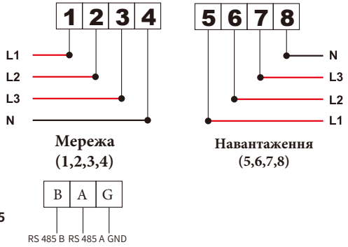
Рис. 7.1 Лічильник Eastron
