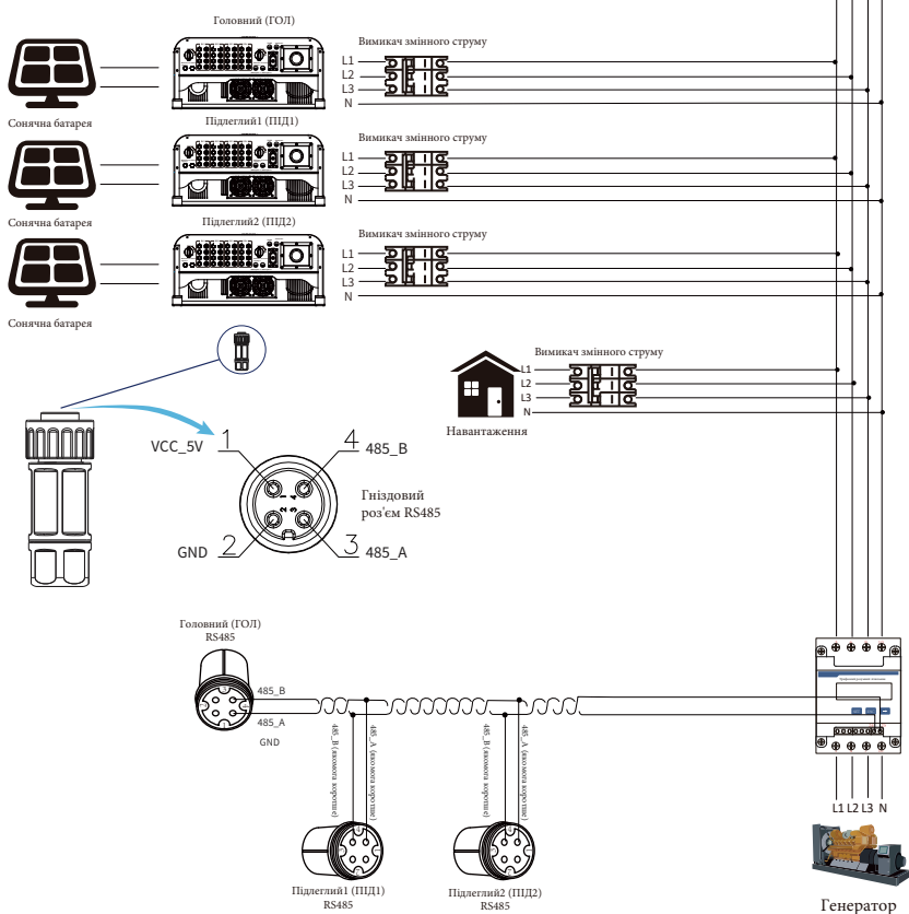
Рис. 7.31 Схема підключення CHNT (таблиця пропускну́ї здатності)
