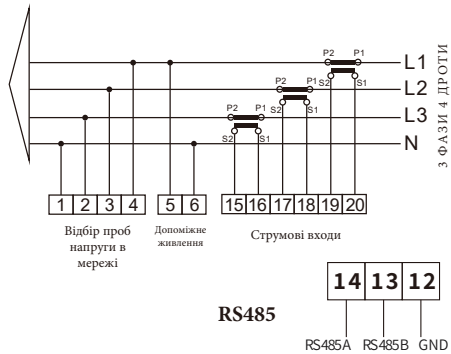
Рис. 7.24 Лічильник Eastron
