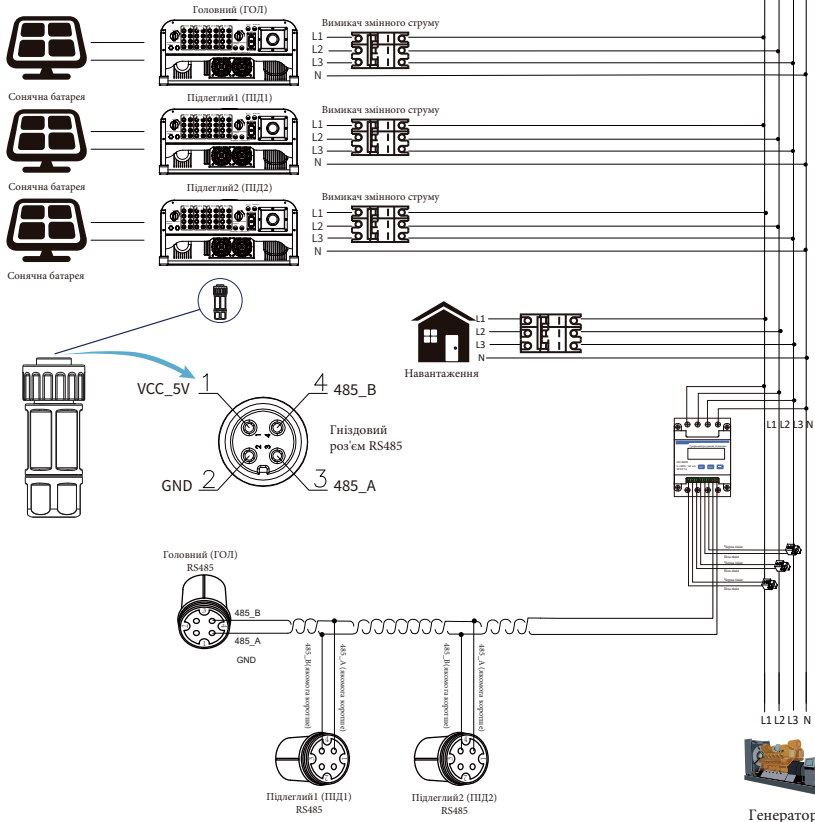
Рис. 7.35 Схема підключення CHNT (таблиця пропускної здатності)
