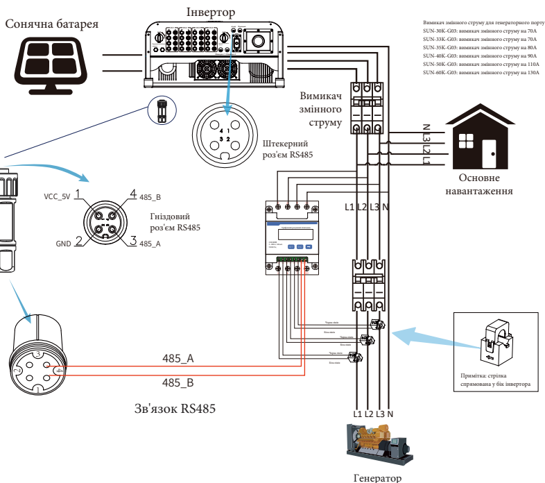
Рис. 7.16 Схема підключення лічильника CHNT
