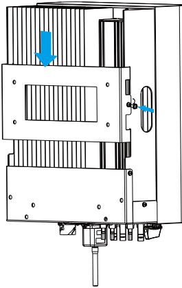
Рис. 4.6 Встановлення інвертора
