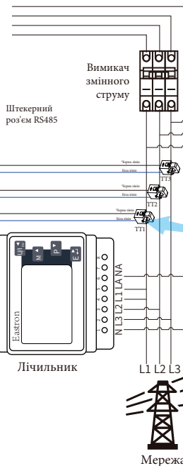
Рис. 7.6 Схема підключення лічильника Eastron
