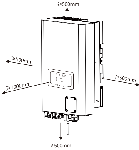
Рис. 4.3 Монтажний проміжок
