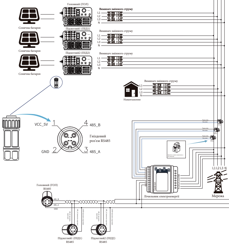
Рис. 7.23 Схема підключення (трифазна електрика)
