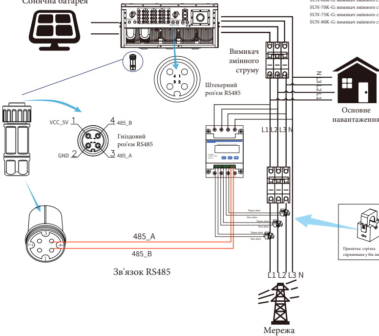
Рис. 7.14 Схема підключення лічильника CHNT
