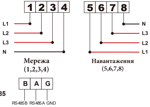
Рис. 7.20 Лічильник Eastron
