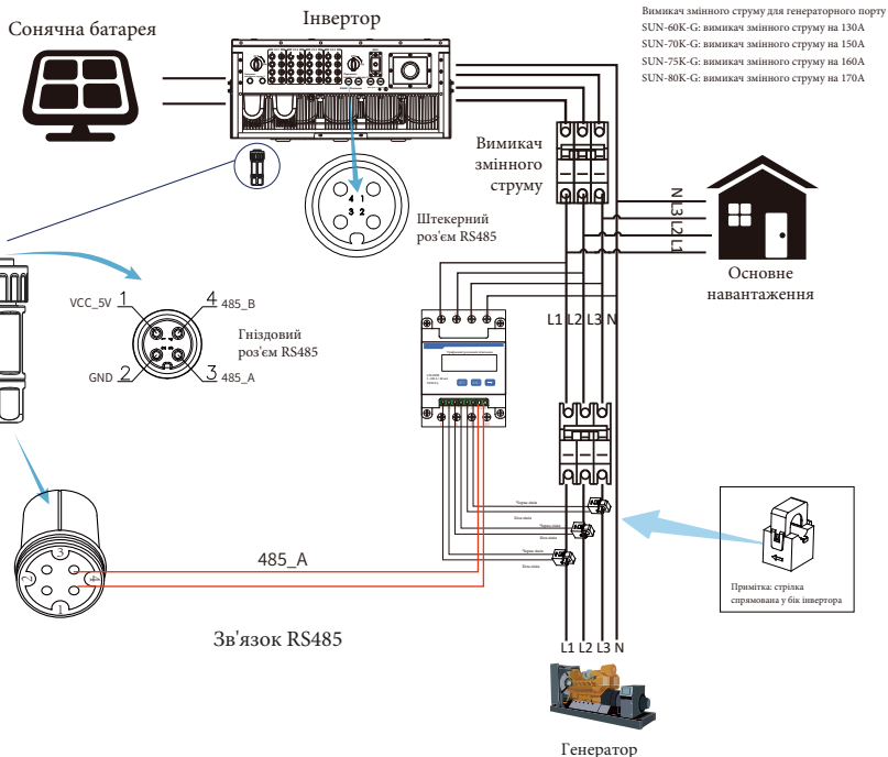
Рис. 7.16 Схема підключення лічильника CHNT
