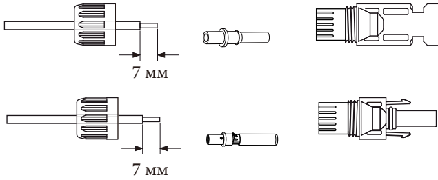
Рис. 5.3 Розбирання накидної гайки роз'єму
