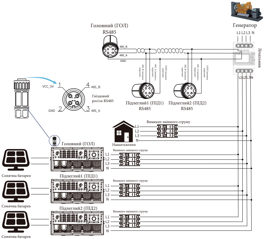
Рис. 7.23 Схема підключення Eastron (таблиця пропускнуної здатності)
