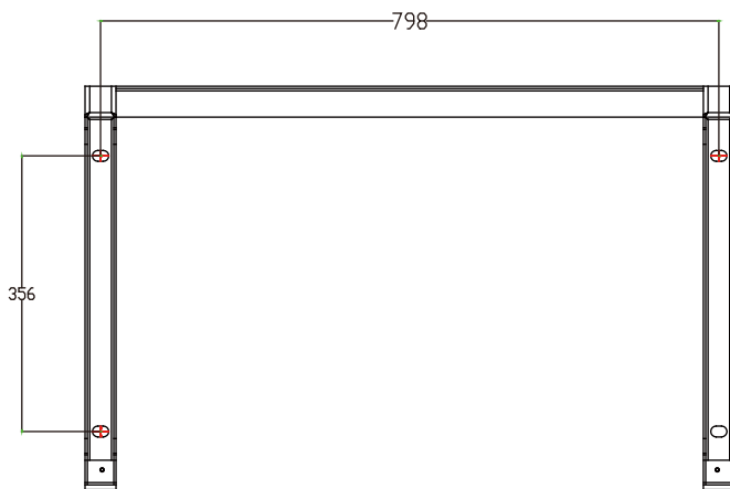
Рис. 4.4 Розміри монтажної кронштейна
