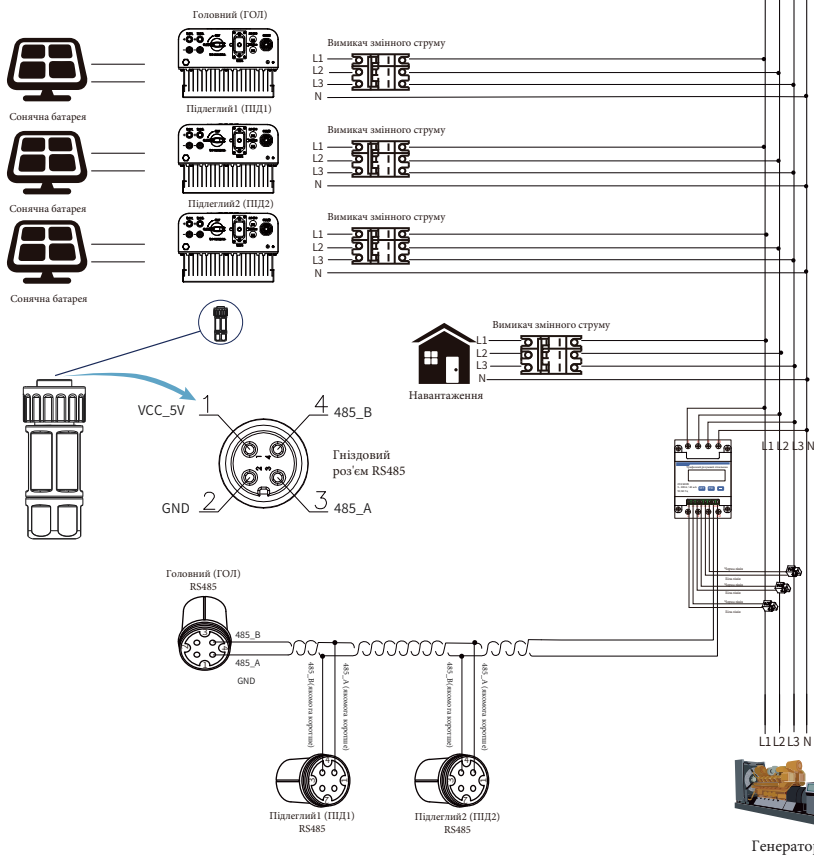
Рис. 7.33 Схема підключення CHNT (таблиця пропускнув здатності)
