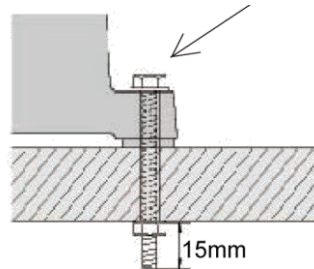
Рисунок 6. Схема фіксації виробу на верстаку.
