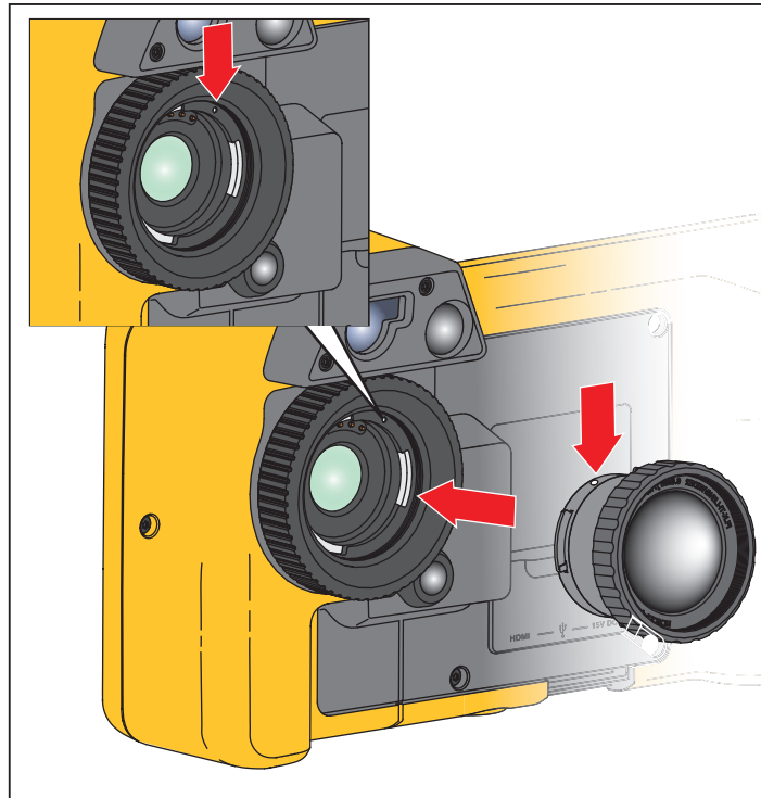
Рисунок 1. Установка дополнительного объектива
