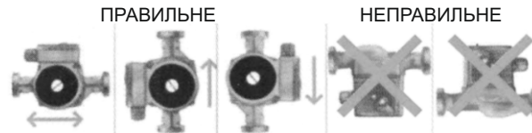
Мал. 3. Установлення насоса.
