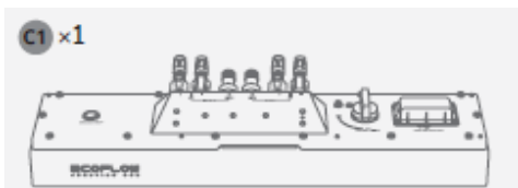
Розподільна коробка акумуляторної батареї
