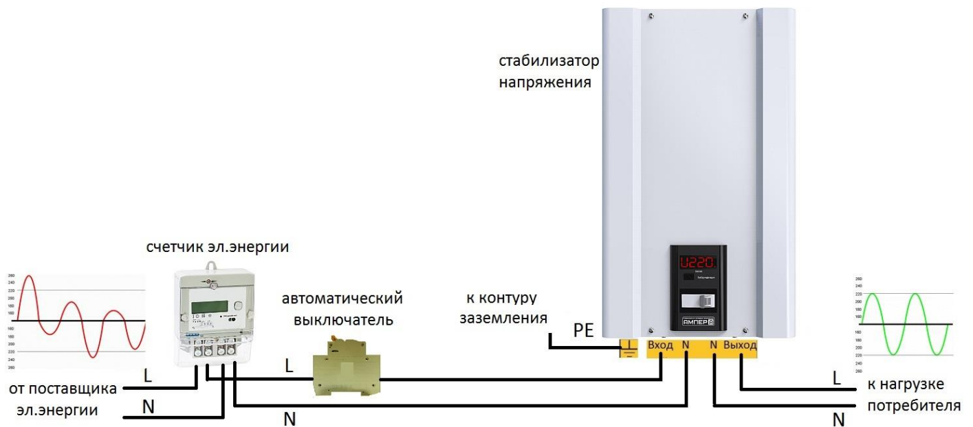
Рисунок 6. Схема подключения стабилизатора к однофазной сети
