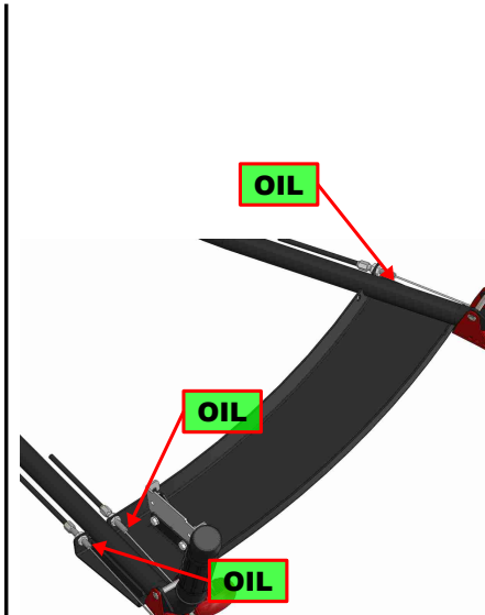
Obr. 7: Mazací místo
