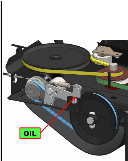
Obr. 6: Mazací místo
